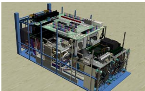
Рис. 1. 3D-модель создаваемого биореактора.
