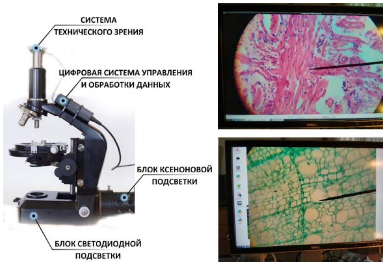
Рис. Лабораторный микроскоп МББ-1А, модификации NZ-M1. Трансляция предметного столика на монитор.
