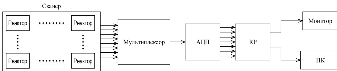
Рис. 4. Функциональная схема сканера
