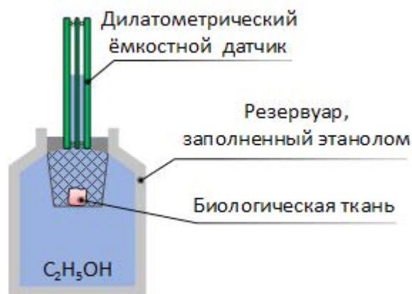
Рис. 2. Устройство для регистрации изменения объема системы образец биологической ткани-этанол
