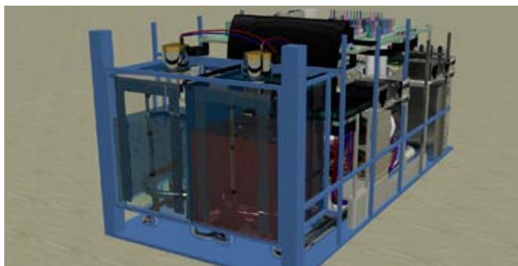
Рис. 1. 3D-модель создаваемого биореактора.
